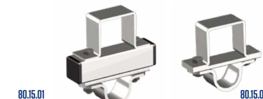
Montagesatz C-Schiene
